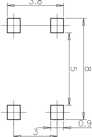
PCB. 焊接图
