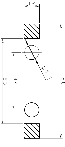
P.C.B. layout
