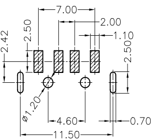
P.C.B LAYOUT(TOL:±0.05)
