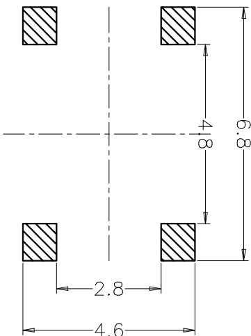
PCB. 焊接图
