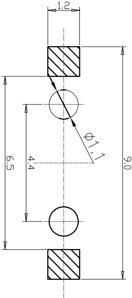
P.C.B. layout
