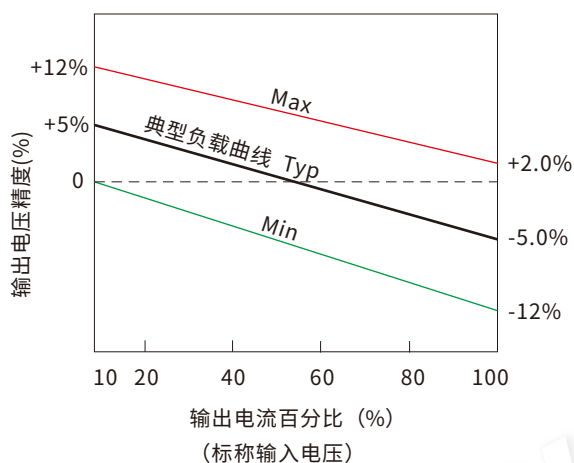
误差包络曲线图 3.3Vdc输出
