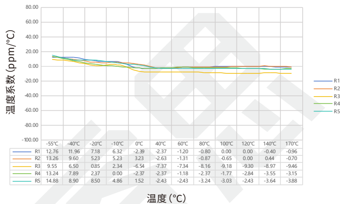
PEWM 系列 4026 规格 0.3mΩ 温度系数实测数据表
