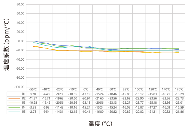
PEWM 系列 4026 规格 0.2mΩ 温度系数实测数据表
