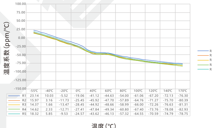
PEWM 系列 4026 规格 1.0mΩ 温度系数实测数据表
