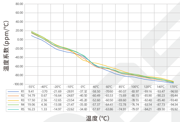
PEWM 系列 4026 规格 0.5mΩ 温度系数实测数据表
