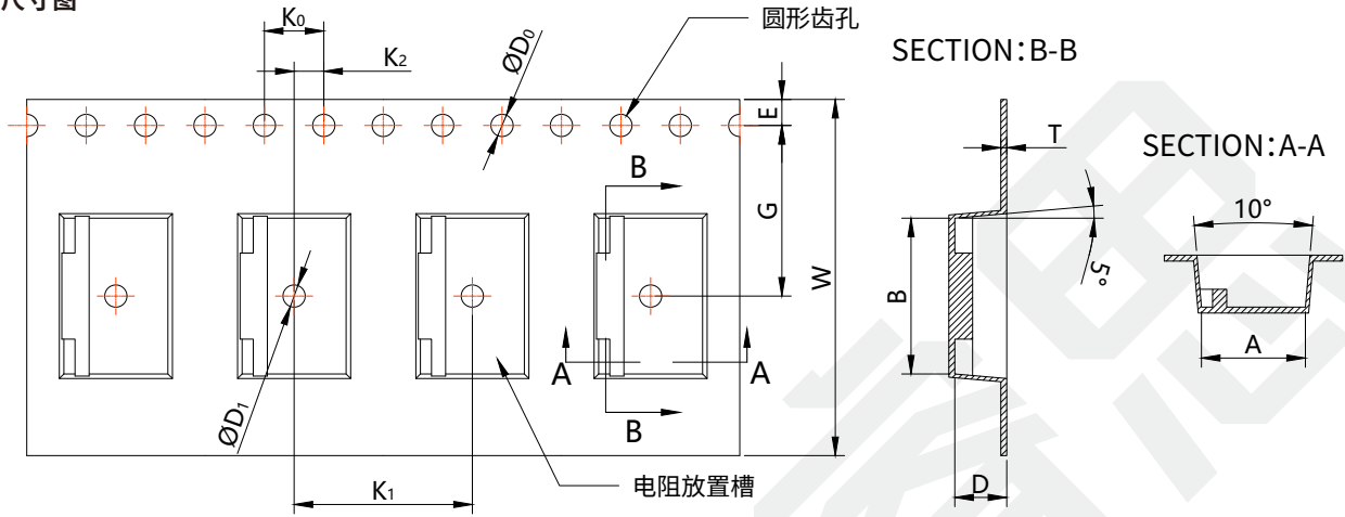
卷编带尺寸图
