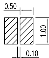
METAL MASK T=0.10 TOLERANCE±0.05(钢网推荐图)
