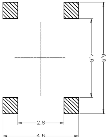
PCB. 焊接图
