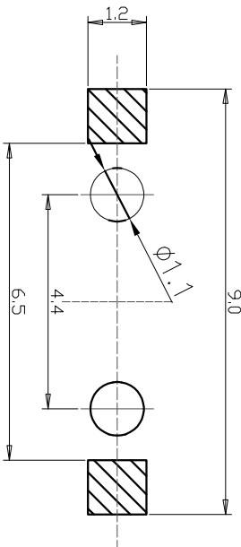
P.C.B. layout
