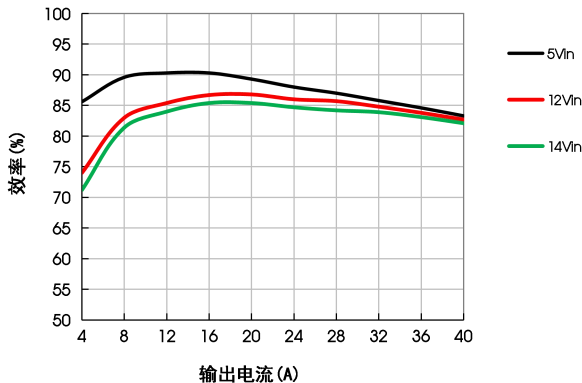
效率Vs输出负载 ( V_{out}=0.6\text{V} )
