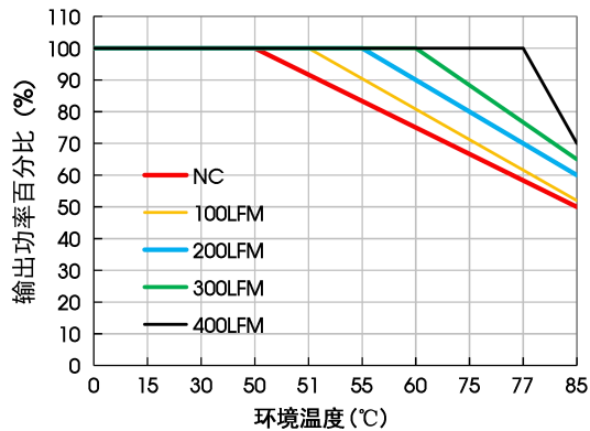
温度降额曲线 (Vo=1.0V)
