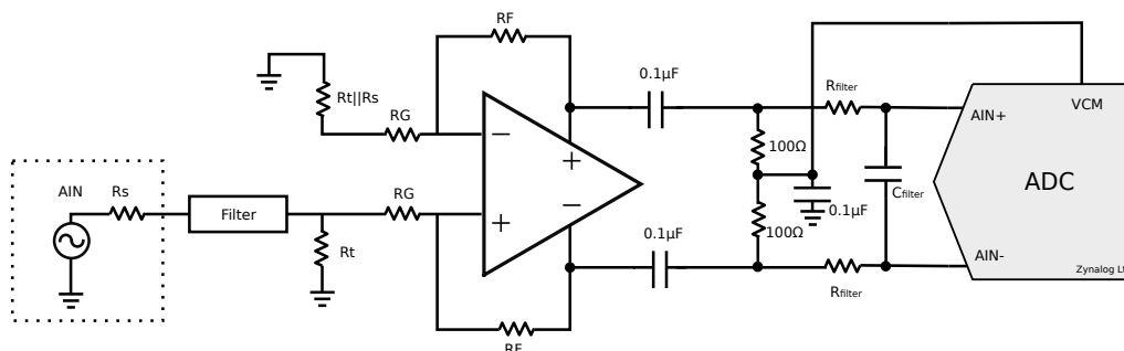
图 7: 使用单端转差分的高速运放的推荐前端电路 (隔离直流信号)
