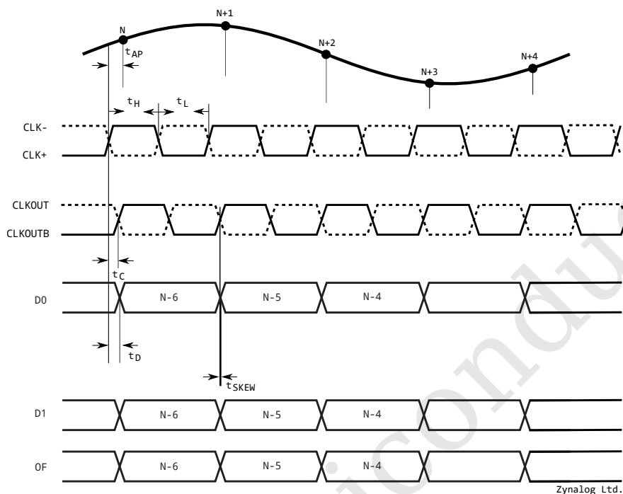
图 3: 数据输出
