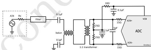
图 6: 输入频率大于第一个 Nyquist Zone 的推荐前端电路
