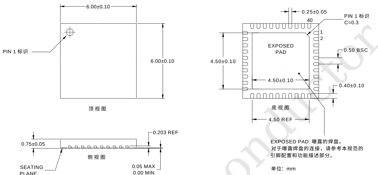
图 13: 封装信息
