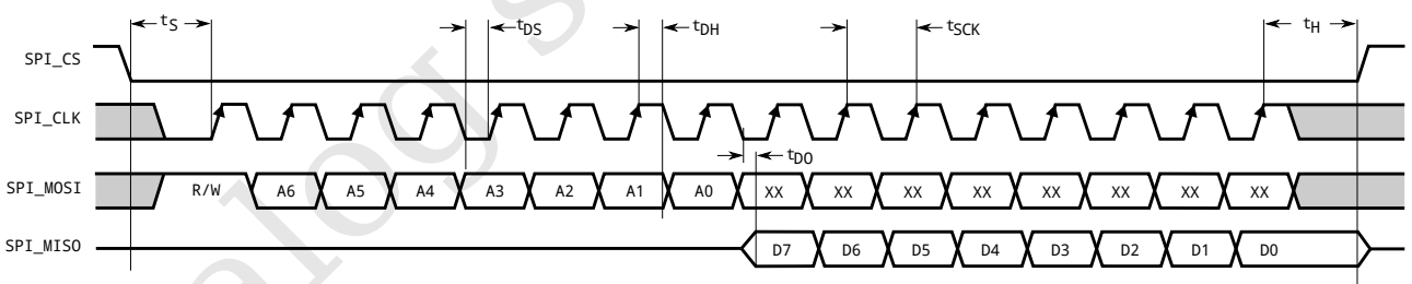
读回时序
