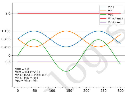
图 4: 输入信号满量程示意图
