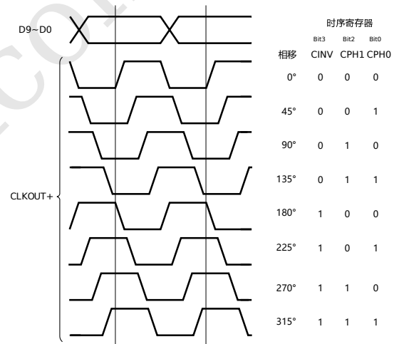
图 11: 相位偏移
