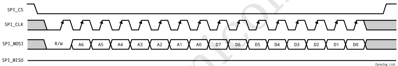
写入时序
