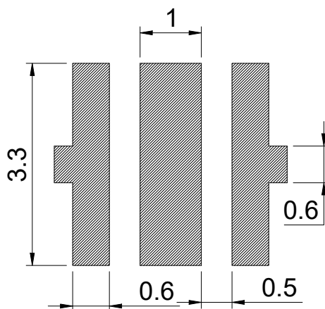
焊盘建议图
