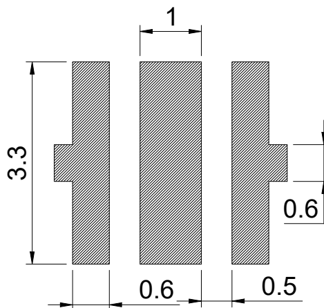
焊盘建议图
