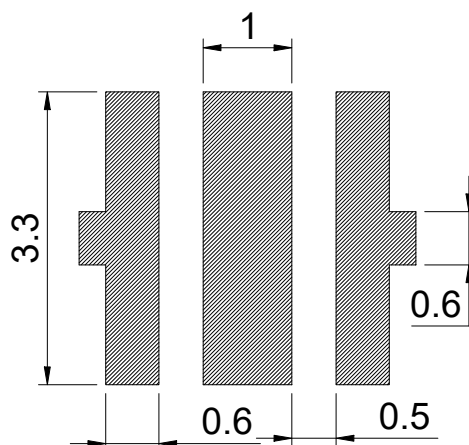
焊盘建议图
