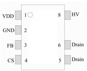
SOP-7 俯视图
