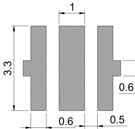
焊盘建议图
