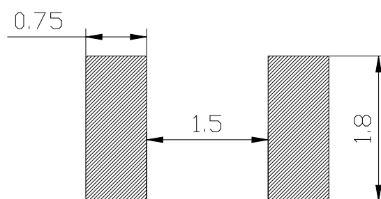
焊盘建议图
