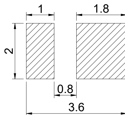
焊盘建议图
