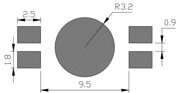
焊盘建议图
