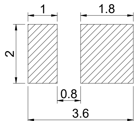
焊盘建议图
