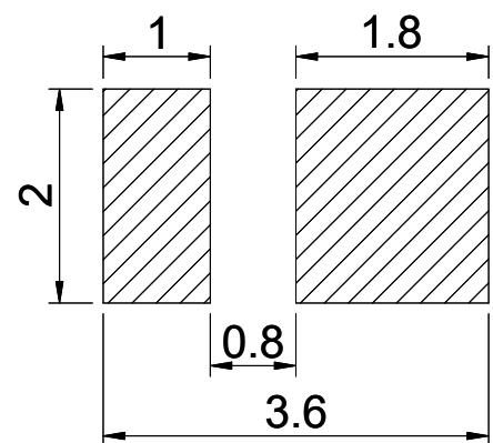
焊盘建议图
