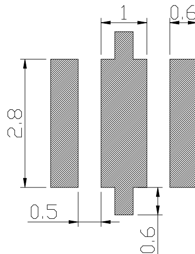
焊盘建议图
