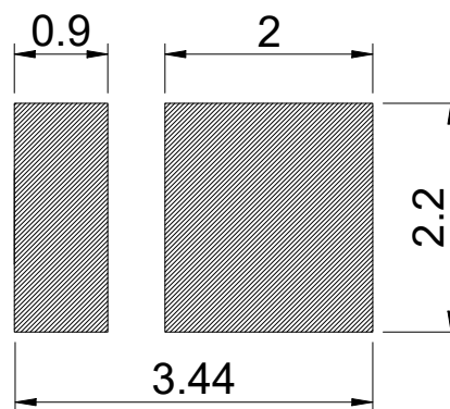
焊盘建议图
