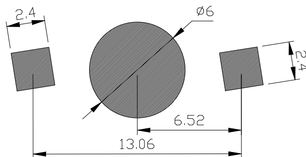
焊盘建议图
