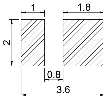
焊盘建议图
