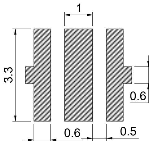
焊盘建议图
