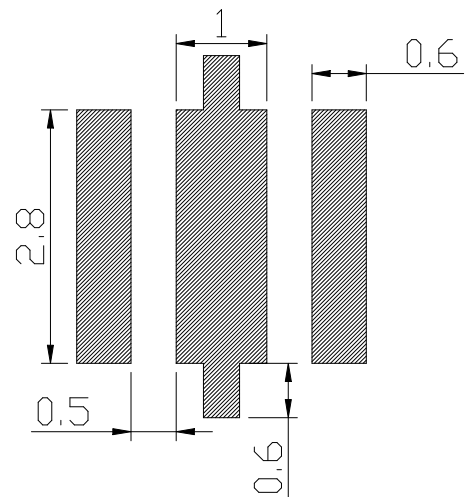
焊盘建议图
