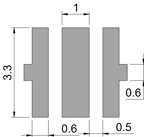
焊盘建议图
