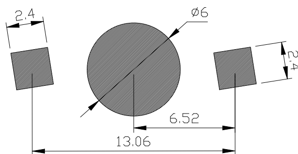
焊盘建议图
