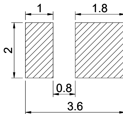
焊盘建议图
