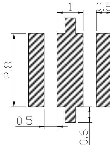
焊盘建议图
