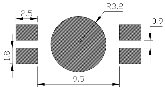
焊盘建议图
