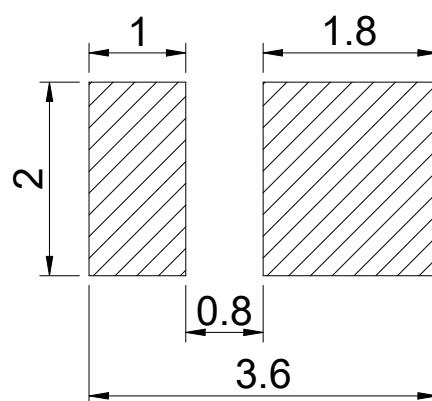
焊盘建议图
