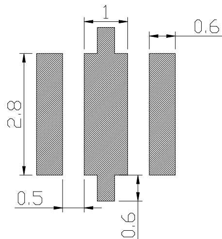
焊盘建议图
