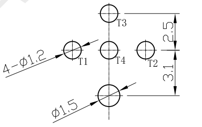
P.C.B LAND DIMENSION
