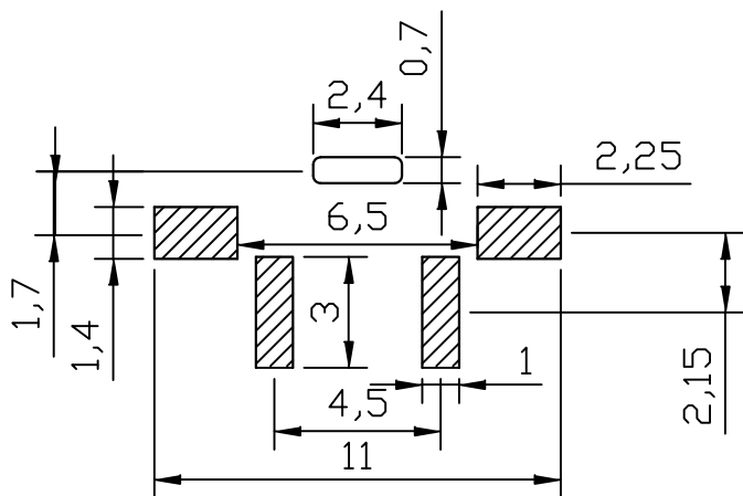
焊接图
