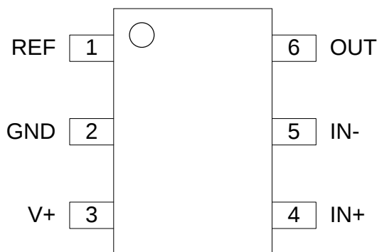
INA21X 引脚排列图
