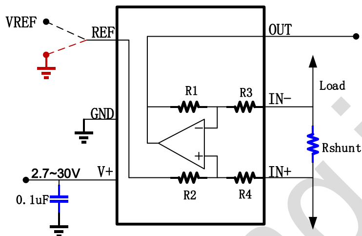
INA21X 功能框图
