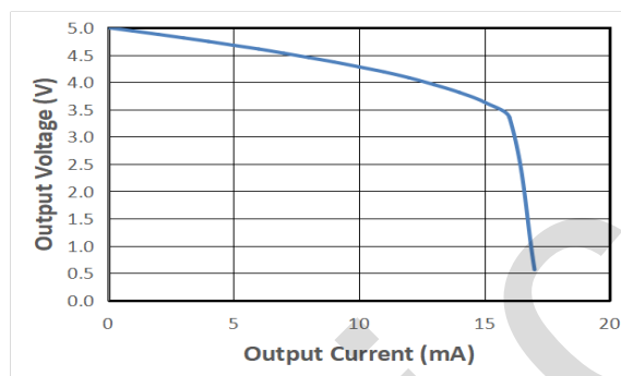
高电平驱动能力
