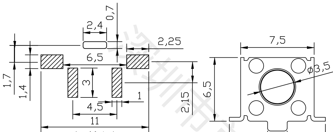
焊接图
