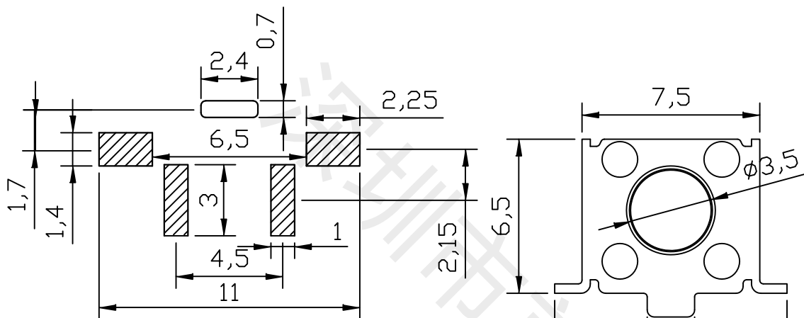
焊接图
