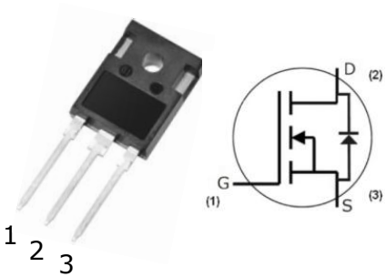
TO-247-3L
