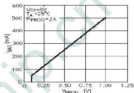
充电电流与 PROG 引脚电压的关系曲线
