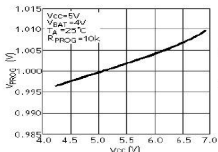
恒定电流模式下 PROG 引脚电压与电源电压的关系曲线
