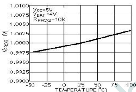
PROG 引脚电压与温度的关系曲线
