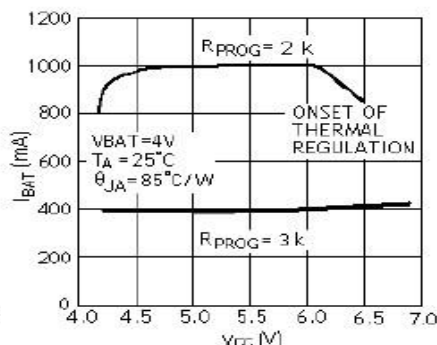
充电电流与电源电压的关系曲线
