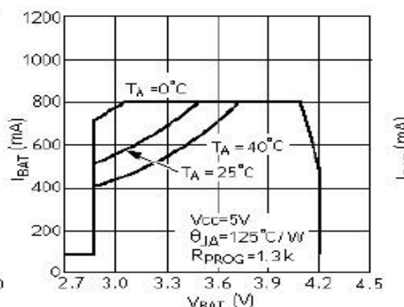
充电电流与电池电压关系曲线
