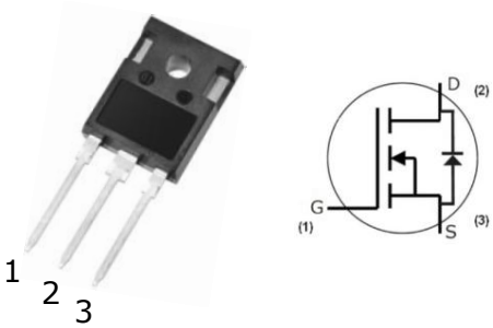
TO-247-3L
