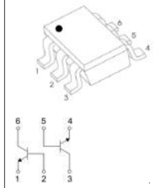
SOT-363
