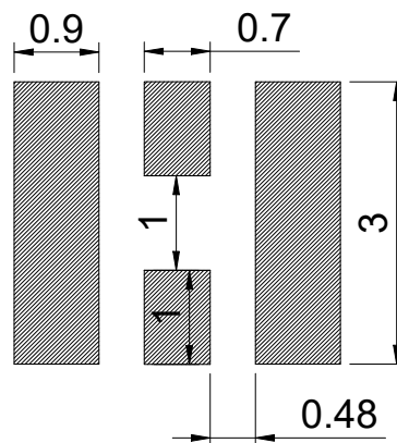
焊盘建议图
