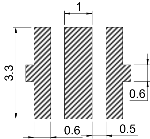
焊盘建议图
