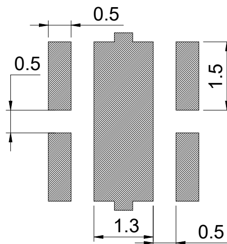
焊盘建议图
