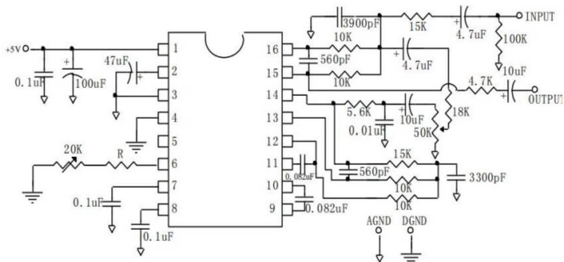
PT2399回音应用电路图
