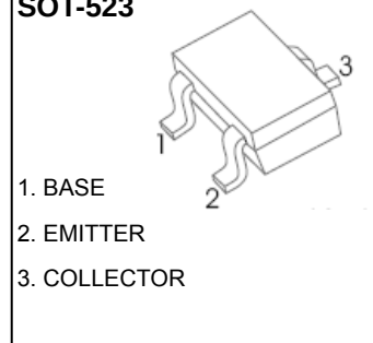
SOT-523
