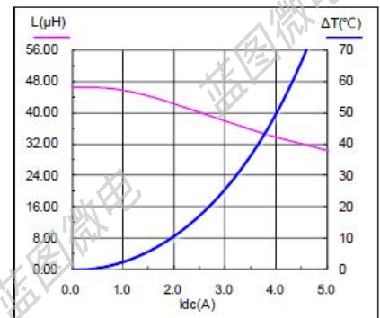
SMS1050-470M
