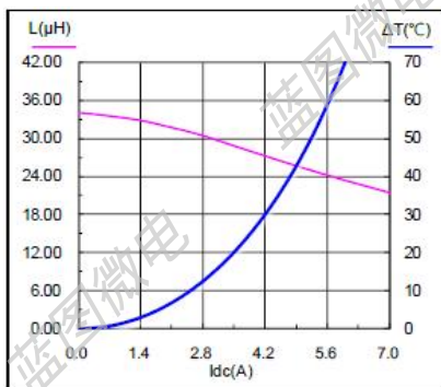
SMS1050-330M
